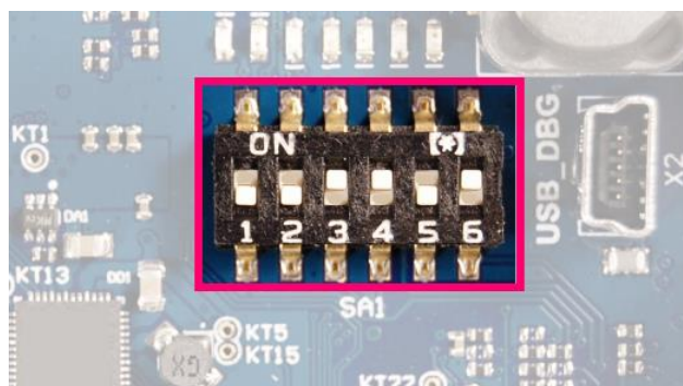
Рис. 3.3. Рабочее положение переключателей.
